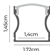
DESENHO TÉCNICO
